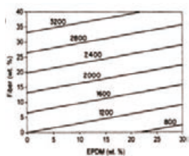
a) Módulo de tração (MPa)
