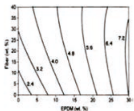
Figura 6 Curvas de níveis em função da composição do compósito.
