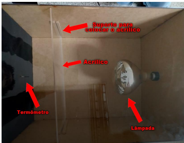
Figura 1: Vista superior do experimento que simula o efeito estufa Fonte: dos autores
